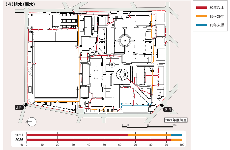
(図2-32) 排水(雨水)配管の経年状況
