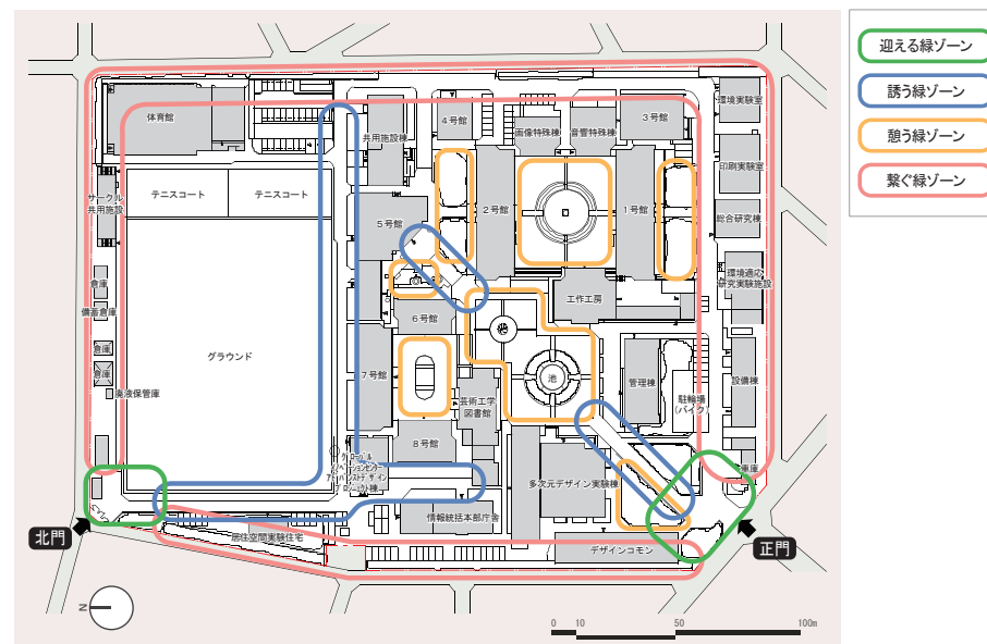
(図3-8) 緑地・植栽帯のゾーニング計画
