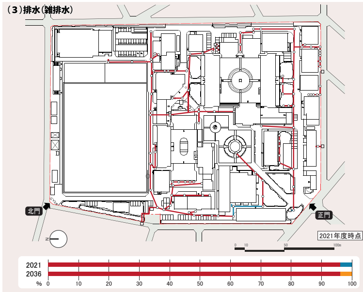
(図2-31) 排水(雑排水)配管の経年状況
