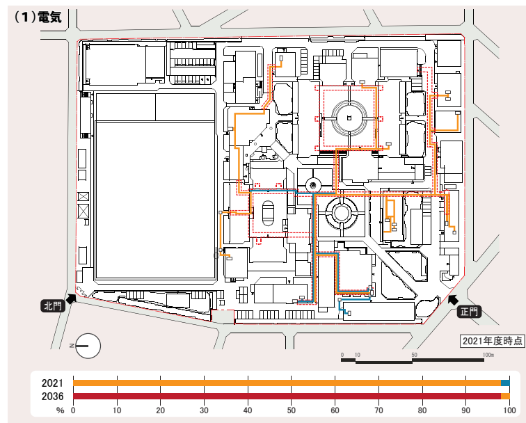
(図2-29) 電気配線の経年状況
