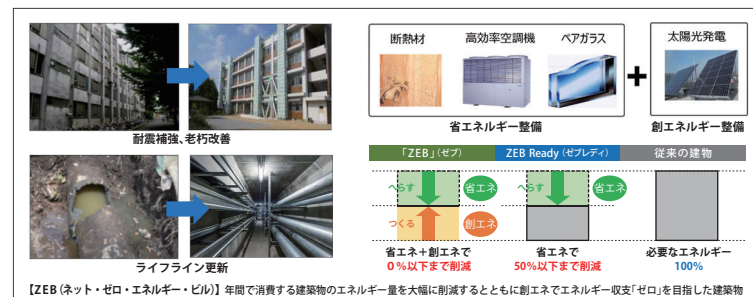
(図3-16)事業イメージ
