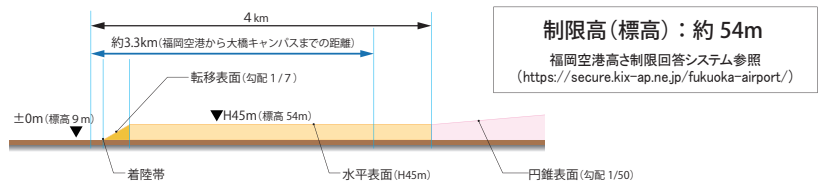
(図2-8) 航空法による高さ制限-1
