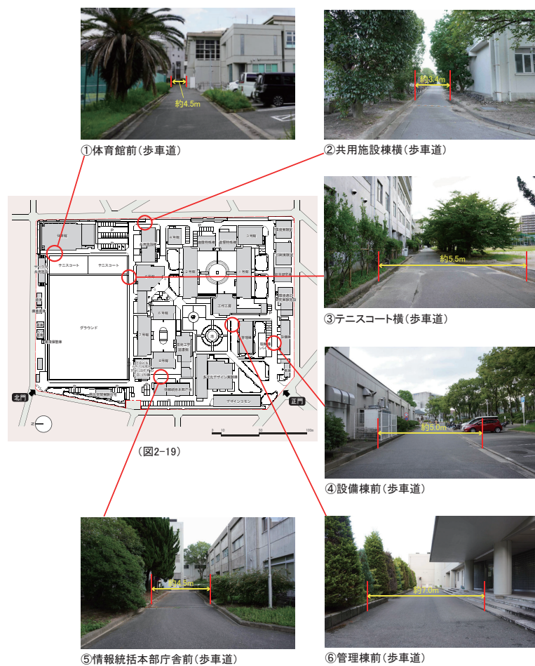
(写真2-16)既存道路の幅員および構成
