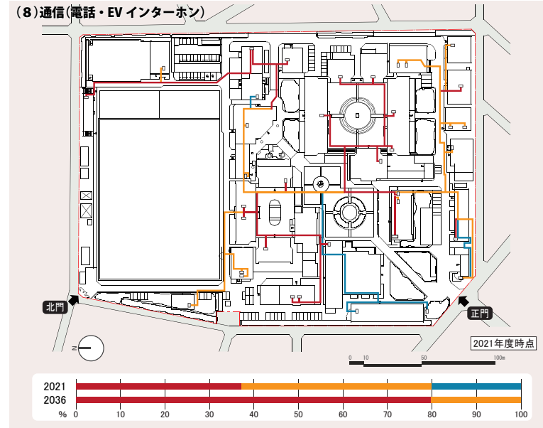
(図2-36)通信(電話・EVインターホン)配線の経年状況
