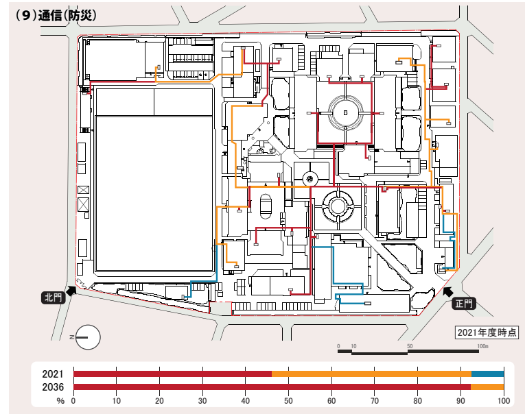
(図2-37)通信(防災)配線の経年状況
